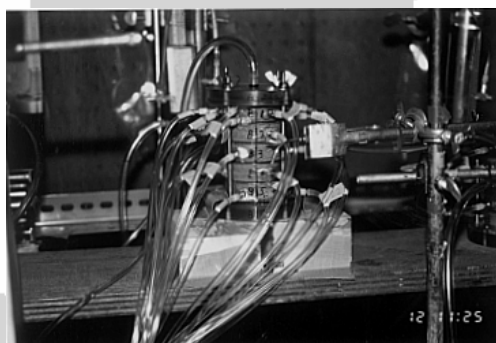
微生物が透水性の及ぼす影響実験
